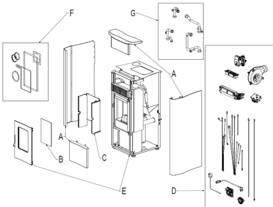
Fig. 1 - Dibujo explotado
